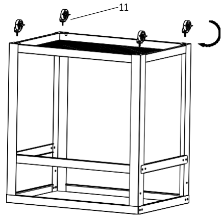
6. M6 4PCS
