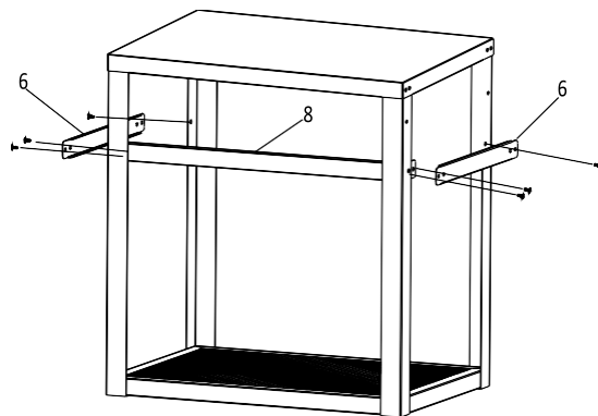
5. A M6*15 2PCS
